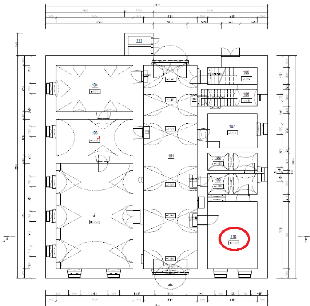
PŮDORYS 1.NP M 1:100
